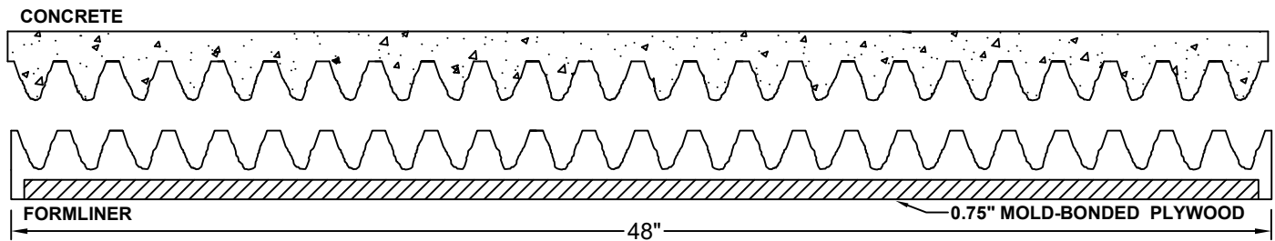
SECTION A-A
