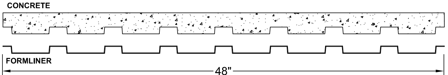
SECTION A-A
