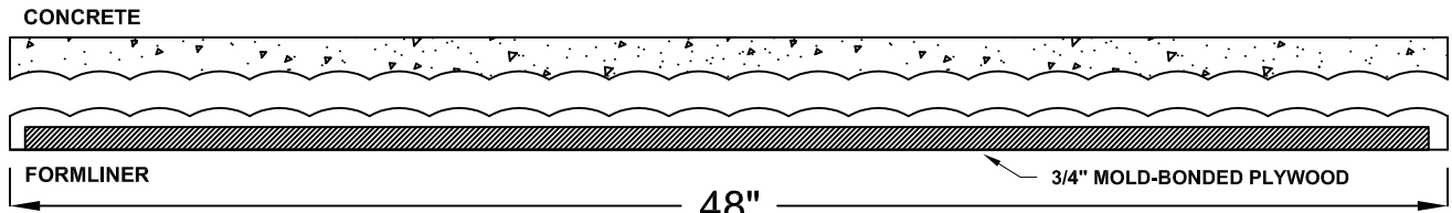
SECTION A-A
