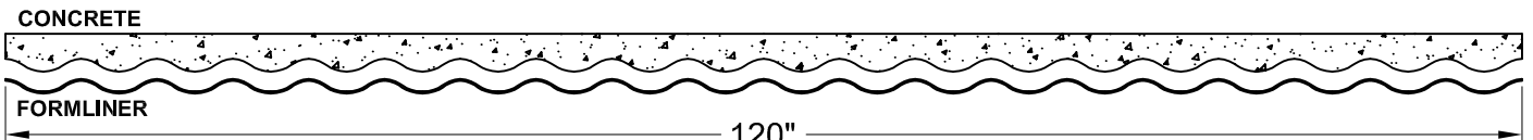
SECTION A-A
