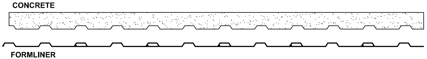
SECTION A-A
