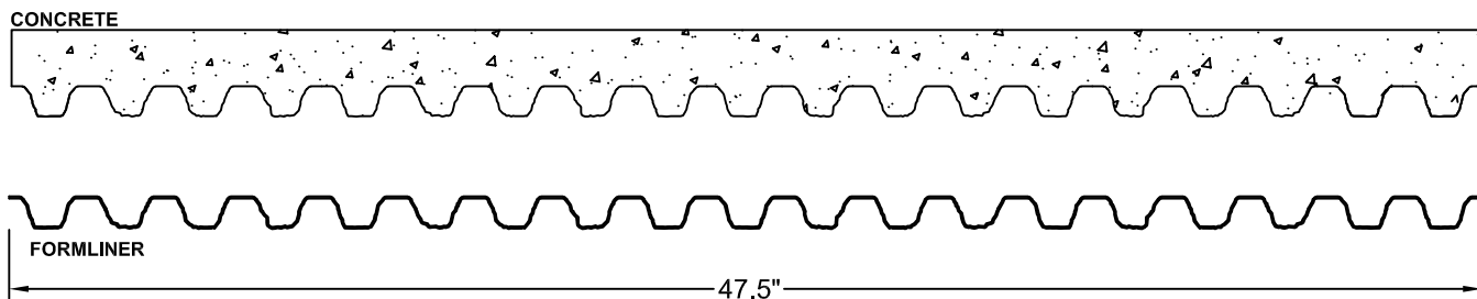
SECTION A-A
