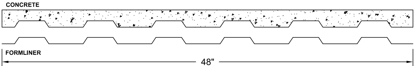
SECTION A-A
