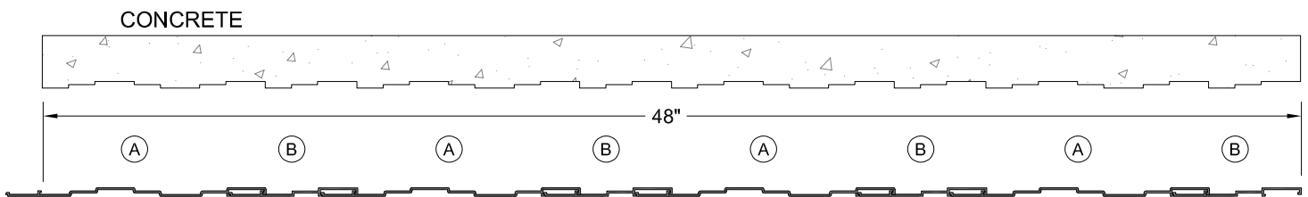
SECTION A-A
