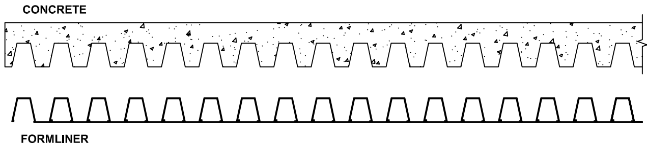
SECTION A-A
