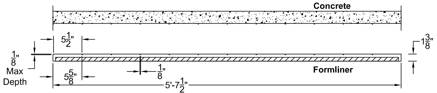
Section A-A
