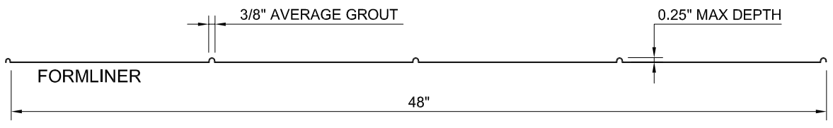
SECTION A-A
