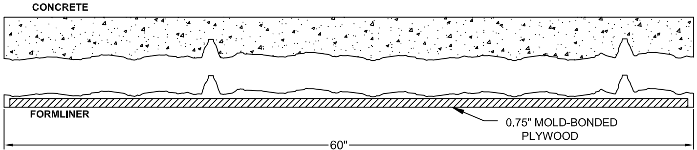
Section A-A
