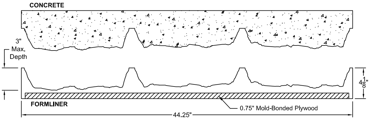
SECTION A-A
