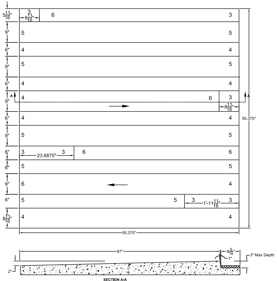
SECTION A-A
