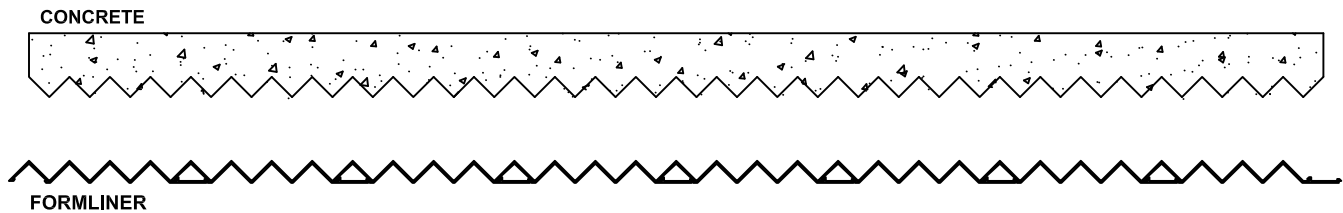
SECTION A-A
