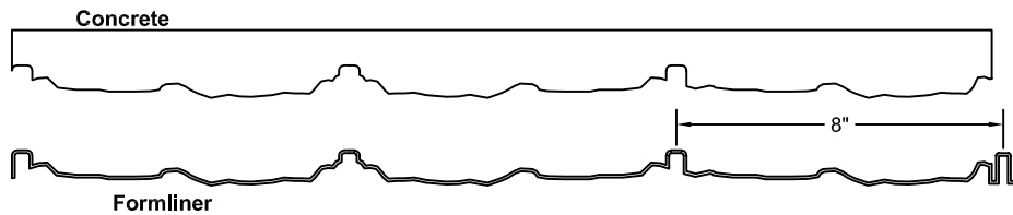
Section A-A
