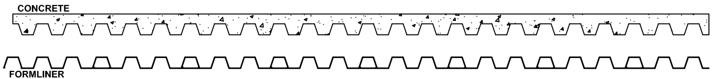
SECTION A-A
