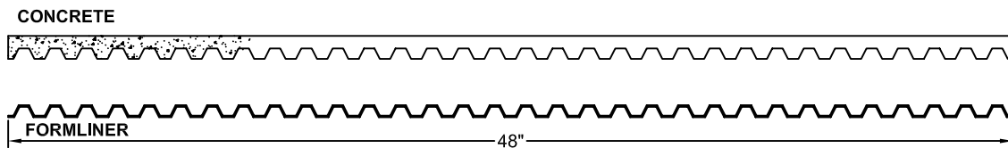
SECTION A-A
